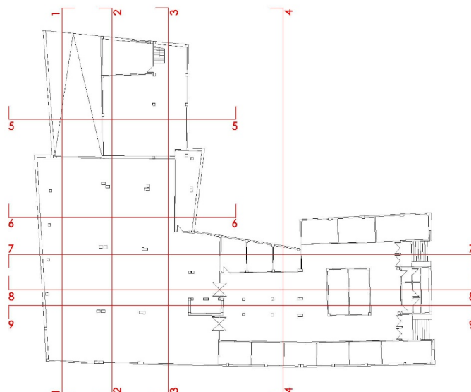
PLANTA SEMISÓTANO
